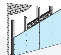
Trasdoso autoportante Knauf W62
